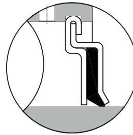
Vedação F + HB
