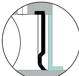
Vedação SLINGER
