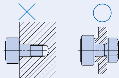
Fig. 4 Métodos de montagem
