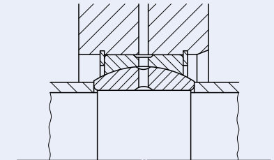
Fig. 10 Exemplos de montagem
