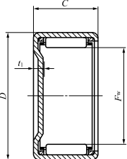
BAM
