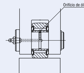
Fig. 2 Posição do orifício de óleo e da direção da carga
