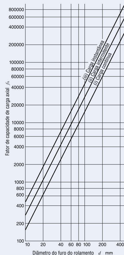
Fig. 1 Fator de capacidade de carga axial
