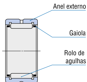
Estrutura do Rolamento de Agulha Tipo Usinado C-Lube
