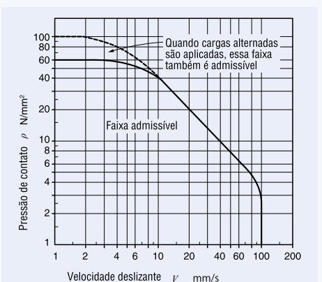
Fig.1 Diagrama pV das buchas esféricas lubrificáveis
