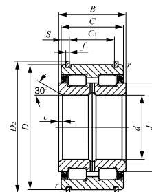
NAS50...UUNR
