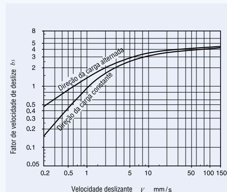
Fig. 4 Fator de velocidade de deslize para Terminais de Rótula tratados com lubrificação
