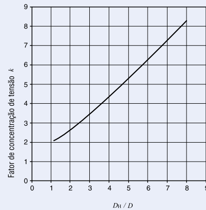
Fig. 7 Fator de concentração de tensão
