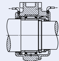
Fig. 23 Lubrificação por circulação de óleo
