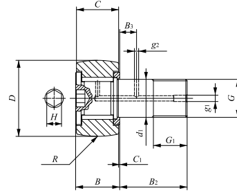
CRH...VBR
