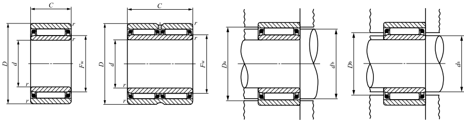
NAF
