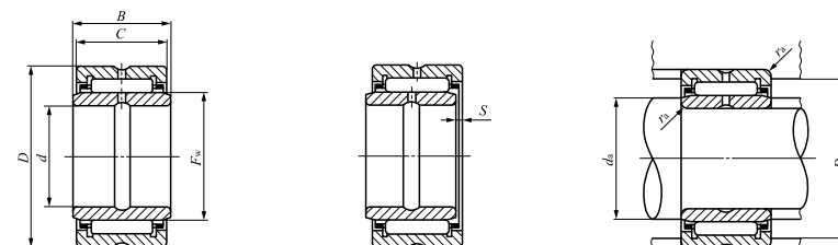
BRI
