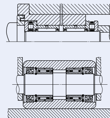
Fig.1 Exemplo de montagem
