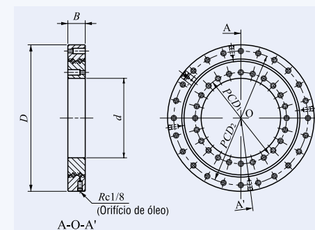
Fig. 5 Exemplo de fabricação
