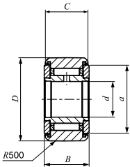
NART...FUUR
