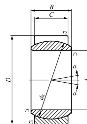
GE...EC
