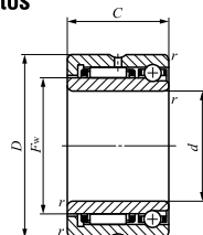
NATA59
