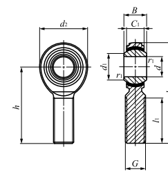
POS...EC
