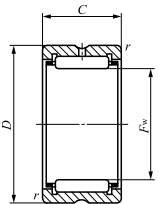
TAF.../SG ( F_w > 26 )
