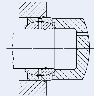
Fig. 9 Método de montagem
