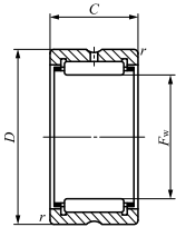
RNA49 RNA48
