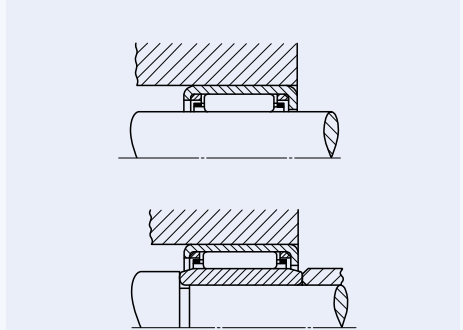
Fig.2 Exemplos de montagem
