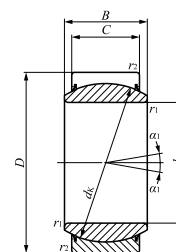
GE...EC-2RS
