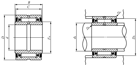
BRI...UU
