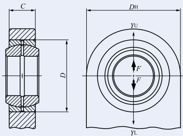
Fig. 6 Formato do alojamento
