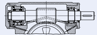
Fig. 22 Lubrificação por respingo de óleo lubrificante
