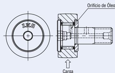
Fig. 2 Posição do orifício de óleo e direção do carregamento
