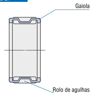
Estruturas das Gaiolas de Agulha para Bielas do Motor
