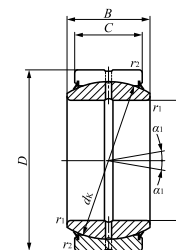
GE...ES-2RS
