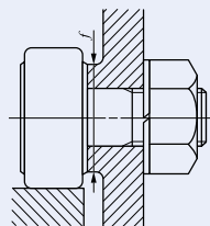
Fig. 1 Superfície de assentamento
