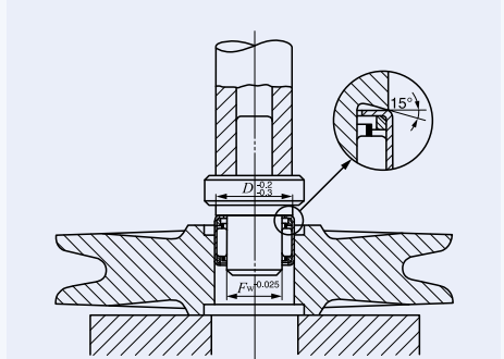
Fig.1 Exemplo de ferramenta de montagem
