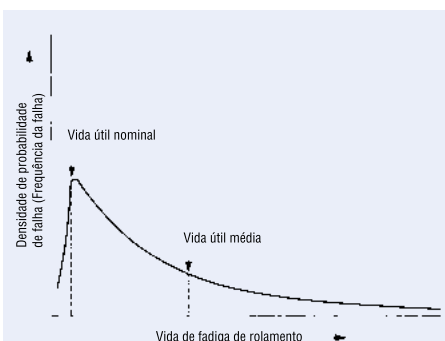
Fig. 1 Variação da vida de fadiga de rolamento
