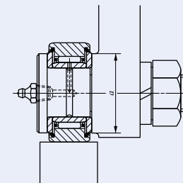
Fig. 1 Dimensão do assentamento correspondente "a"
