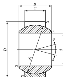
GE...G
