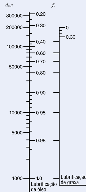
Fig. 2 Fator de correção de velocidade
