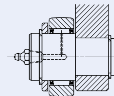
Fig. 3 Exemplo de montagem do Rolo de Apoio sem anel interno
