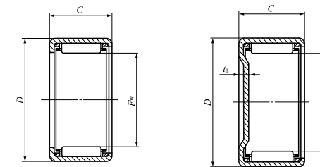
TA...Z
