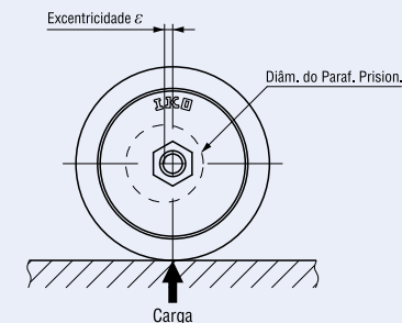
Fig. 5 A posição de referência para ajuste dos Rolos de Comando de Parafuso Prisioneiro Sólido Excêntrico e Rolos de Comando Excêntricos
