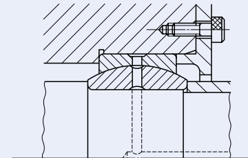
Fig. 10 Exemplos de montagem
