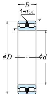
Rolamento Lado Livre Tipo RSF
