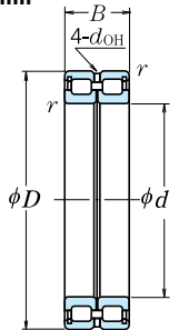
Rolamento Lado Fixo Tipo RS
