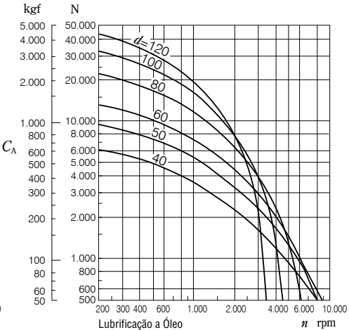
Fig. 5.13 Carga Axial Permissível nos Rolamentos de Rolos Cilíndricos Para rolamentos da série de diâmetro 3 ( k=1,0 ) em carregamento contínuo e lubrificados com graxa ou óleo.
