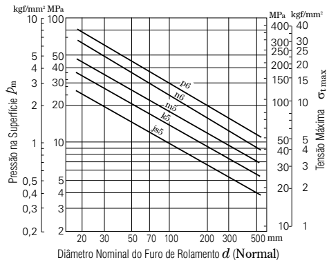
Fig. 15.6 Pressão na Superfície p_m e Tensão Máxima \sigma_{t \max} para a Interferência Máxima dos Ajustes
