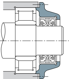
Fig. 11.9 Exemplo de Retentores (2)
