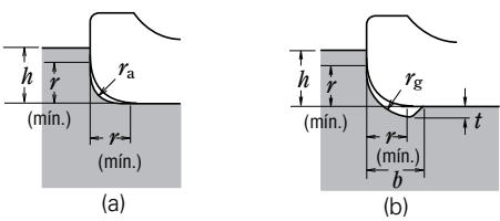
Fig. 11.2 Configuração e Dimensões do Chanfro do Rolamento e Raio de Canto do Eixo
