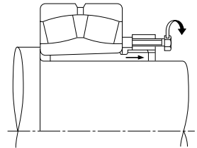
Fig. 14.17 Remoção da Bucha de Desmontagem (2)
