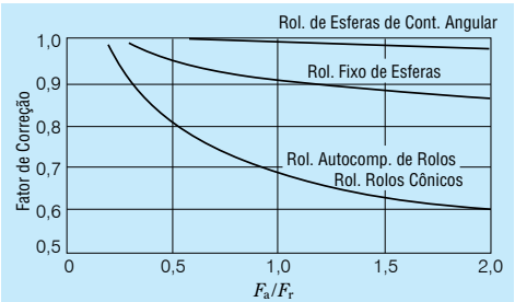
Fig. 6.2 Correção do Limite de Rotação devido à Carga Combinada
